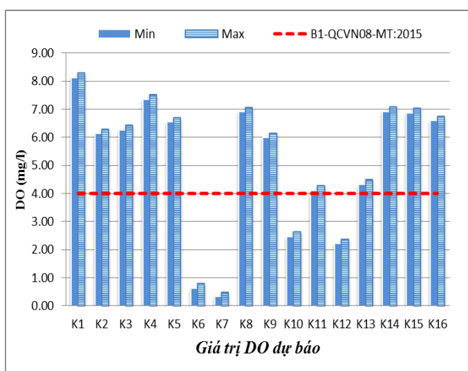
Dự báo hàm lượng DO từ ngày 29/3 – 4/4/2019
