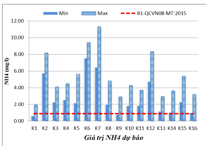
Dự báo hàm lượng \text{NH}_4^+ từ ngày 29/3 – 4/4/2019
